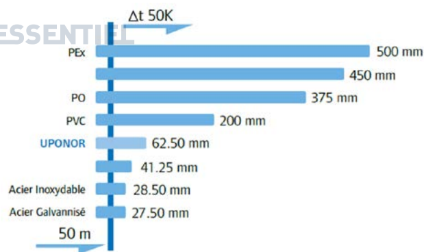
Dilatation thermique de divers matériaux pour un tube de 50 m et \Delta T 50^\circ C
