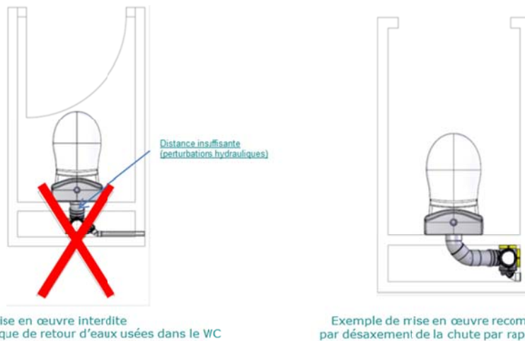
Figure 9 – Recommandation de mise en œuvre en cas d'accolement du WC à la cloison de gaine (valable également pour toute chute destinée à l'évacuation des eaux vannes)
