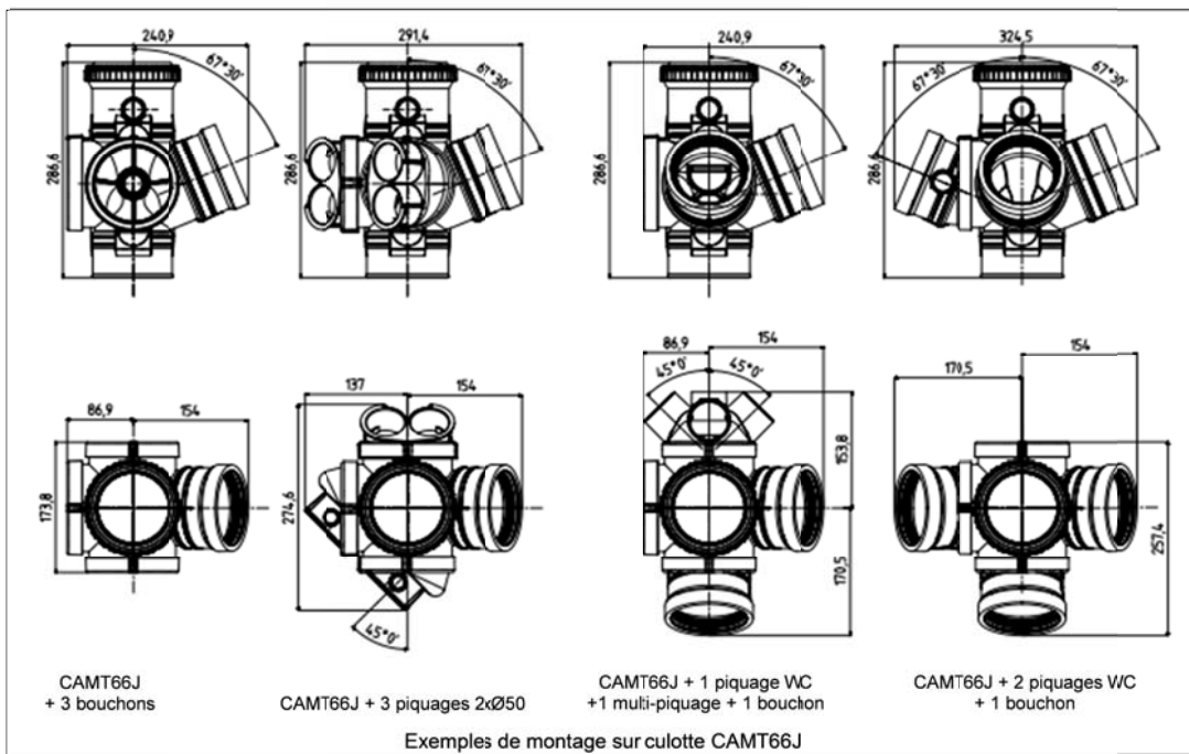
Figure 4 - Cotes d'encombrement des culottes universelles modulaires type Maxicompact®
