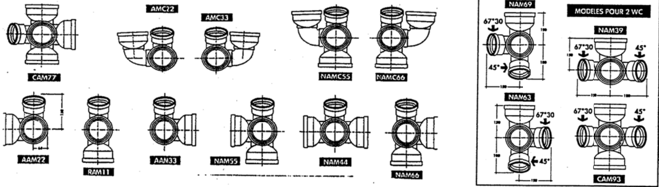
Figure 1 - Culottes avec coude et culottes pour 2 WC
