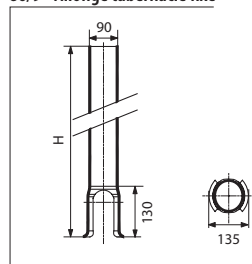
86/9 - Allonge tabernacle fixe
