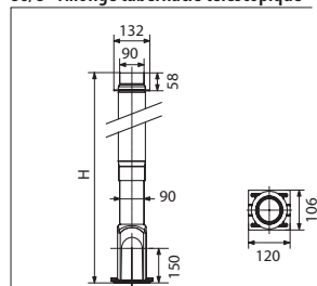
86/8 - Allonge tabernacle télescopique
