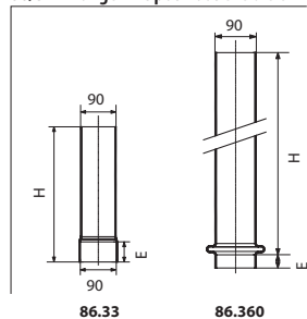
86/3-8 - Tube télescopique
