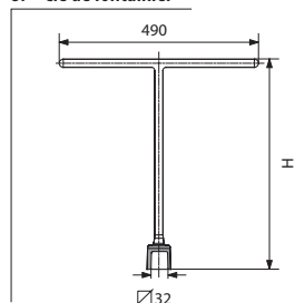
86/3 - Allonge PVC pour bouche à clé
