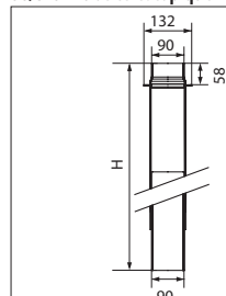
86/8 - Allonge tabernacle télescopique
