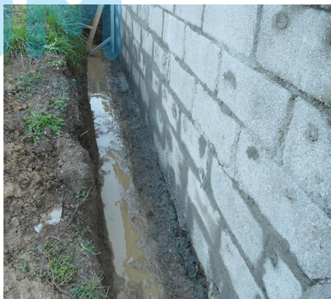
FIGURE N°5 : REJOINTOIEMENT DES PAREMENTS DES FONDATIONS
