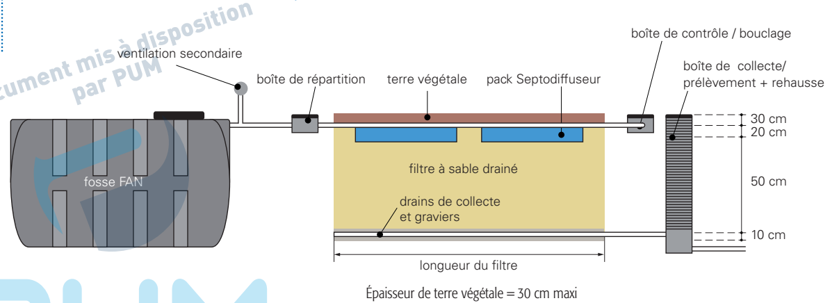
Schéma de la station SEPTODIFFUSEUR SD22 : vue de profil
