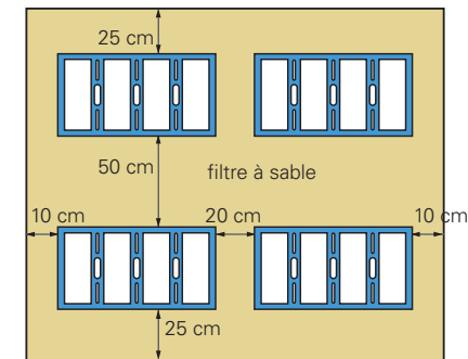
Exemple de répartition des packs SEPTODIFFUSEUR pour une filière SD22
